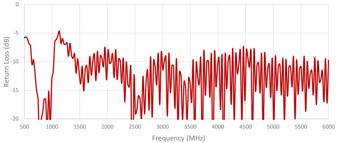
Cable 2: 5GNR
