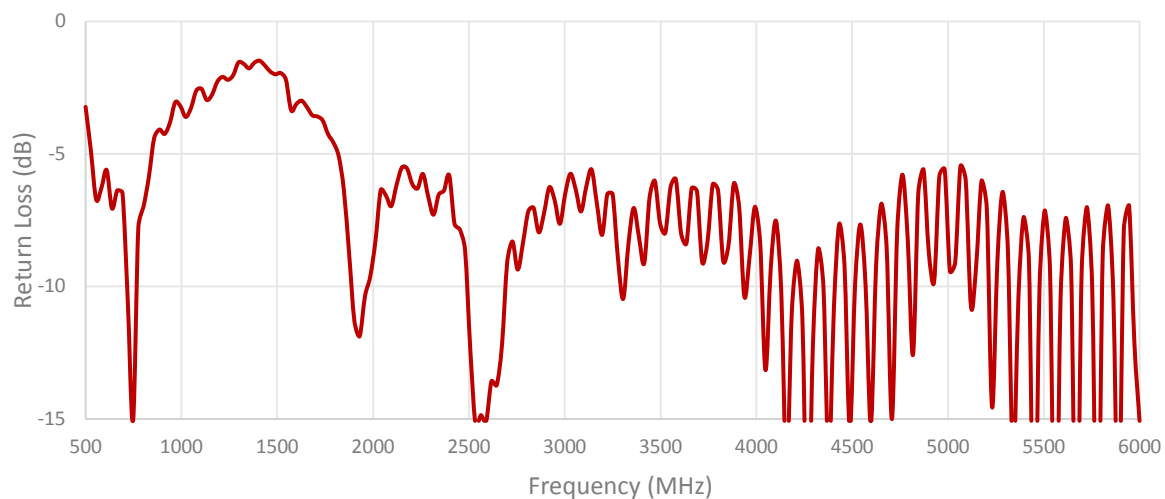
Cable 2: 5GNR
